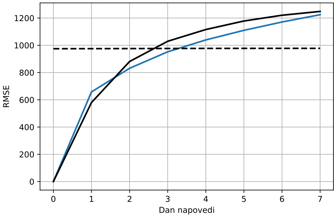
Uspešnost napovedi Z500 - Filtri (2, 4, 8)
